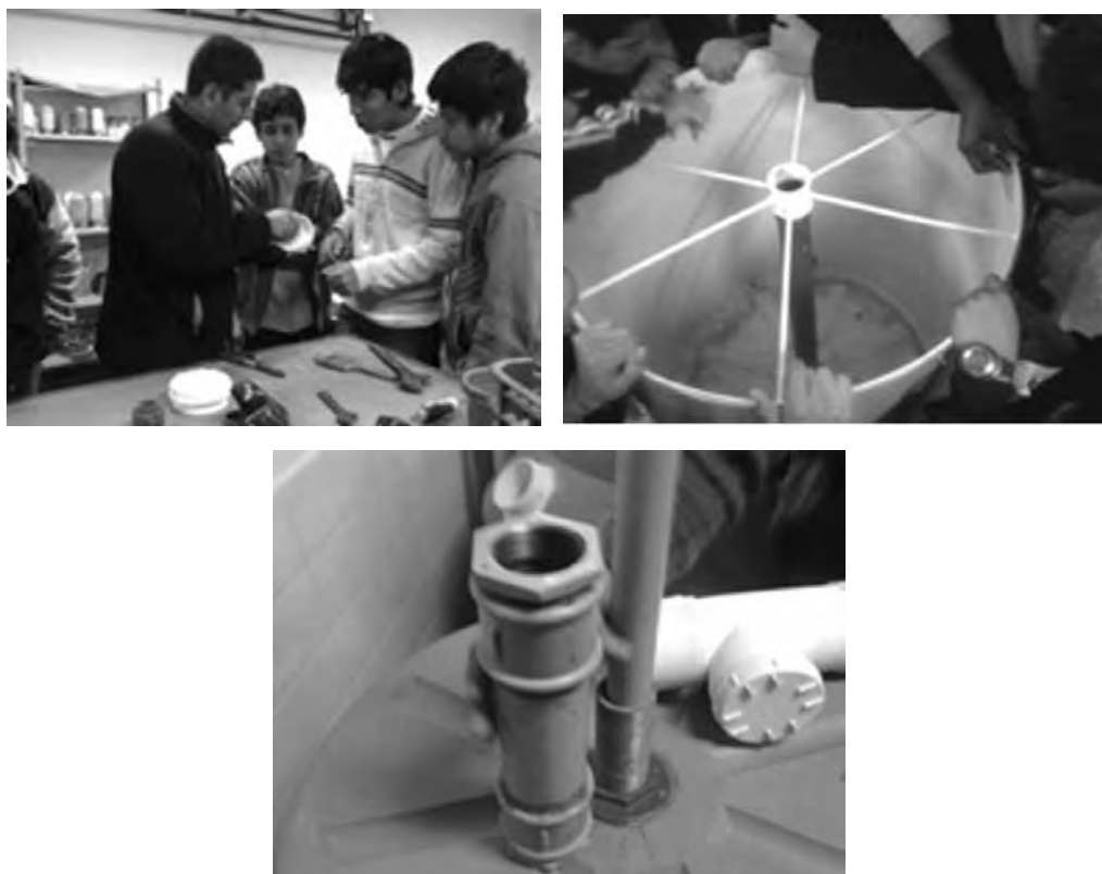
Figs. N° 14, 15 y 16 Construcción biodigestor prototipo-avance, conexiones de entrada y salida
