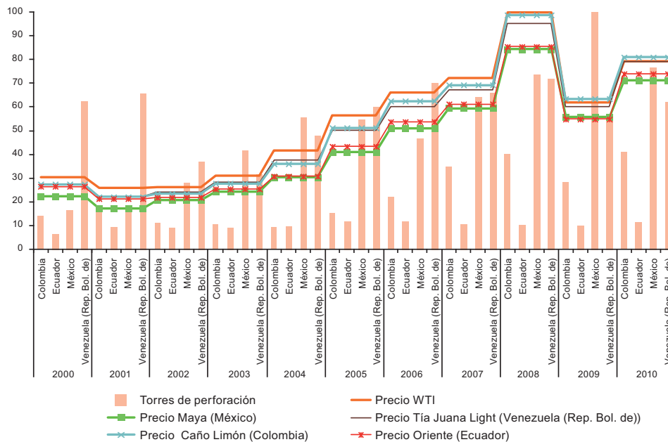
Gráfico A.3 AMÉRICA LATINA (PAÍSES SELECCIONADOS): ACTIVIDADES DE PERFORACIÓN Y EVOLUCIÓN DE LOS PRECIOS DEL PETRÓLEO, SEGÚN TIPO DE CRUDO, 2000-2010 a (En número de torres de perforación y dólares por barril de petróleo)
