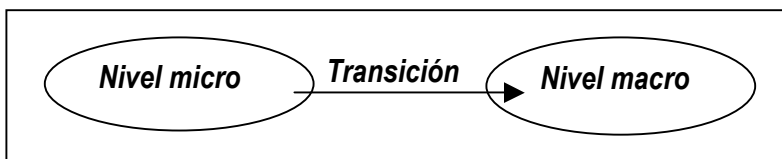
Fig.4 Forma sistémica
